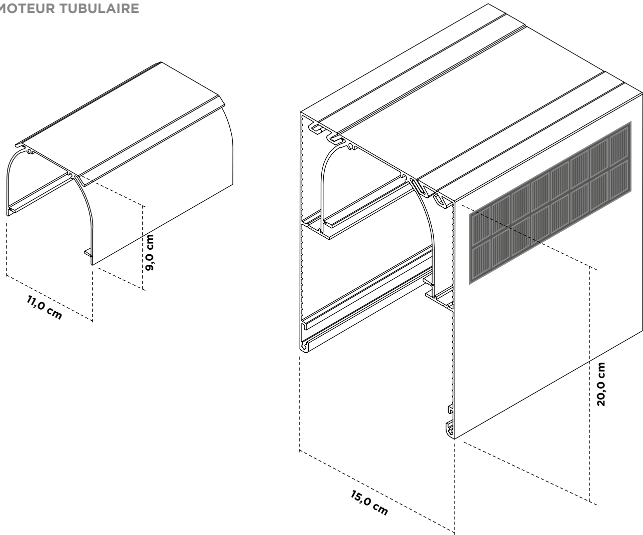
MOTEUR TUBULAIRE
